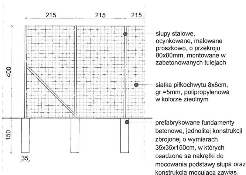
SCHEMAT PIŁKOCHWYTU skala 1:100
