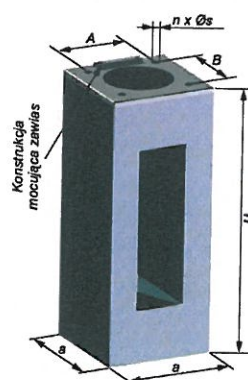
SCHEMAT FUNDAMENTU PREFABRYKOWANEGO skala 1:100
