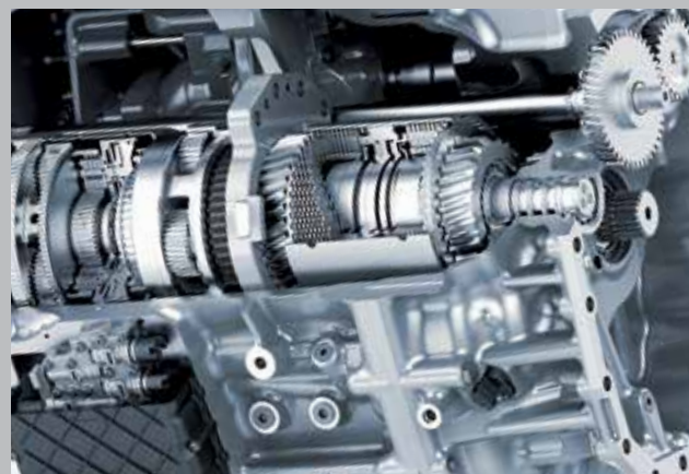
Napęd bezstopniowy TTV umożliwia jazdę z prędkościami od 0 do 40 km/h przy bardzo obniżonej prędkości obrotowej silnika.
